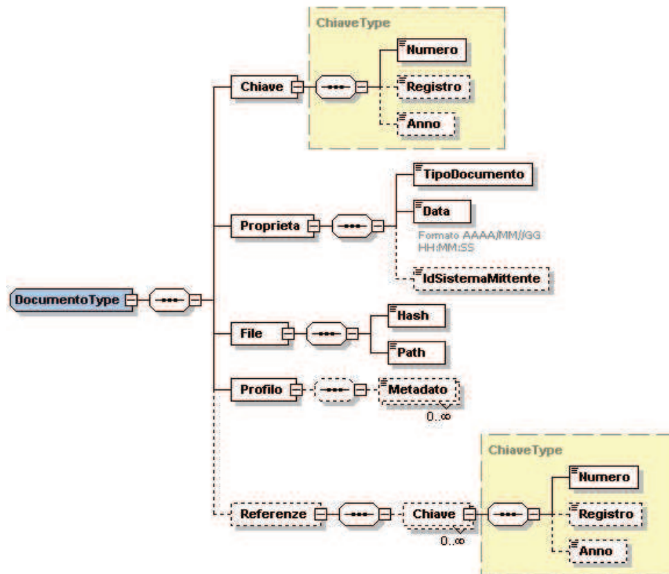
Figura 3 - Nodo documento
